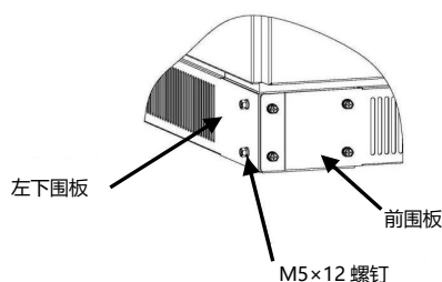
图 6-3 下围板安装
