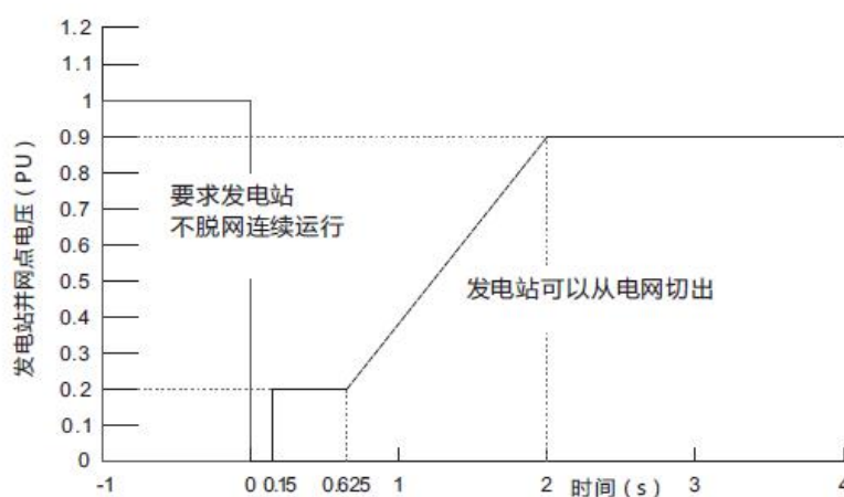
图 4-1 低压穿越曲线
