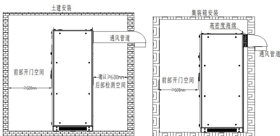
图 5-4 安装空间要求建议
