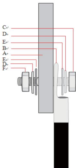
图 6-1 接线端子
