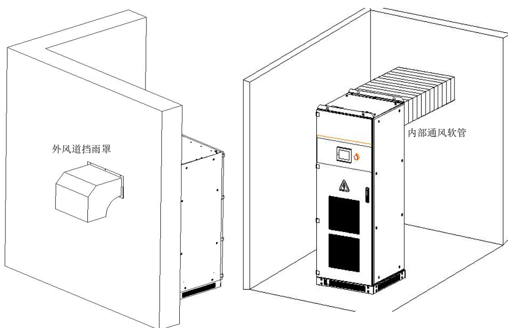
图 5-9 变流器外加风道示意图
