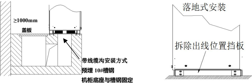
图 5-5 底座安装固定
